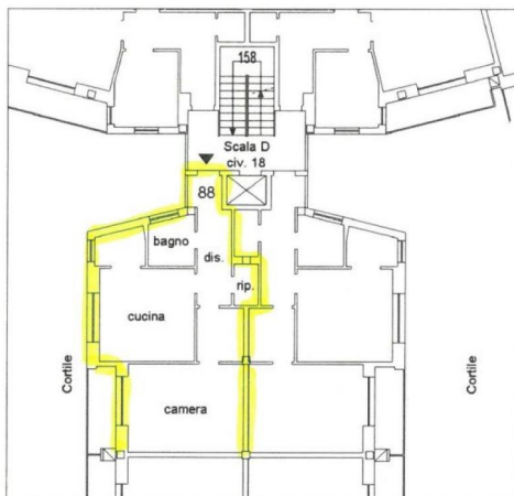
Pianta piano secondo h= 300
